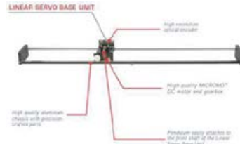
Khối servo cơ bản
